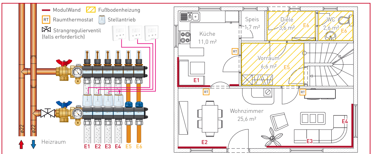
▲ Kombination von Heizsystemen, Beispiel Einfamilienhaus (Erdgeschoß)
