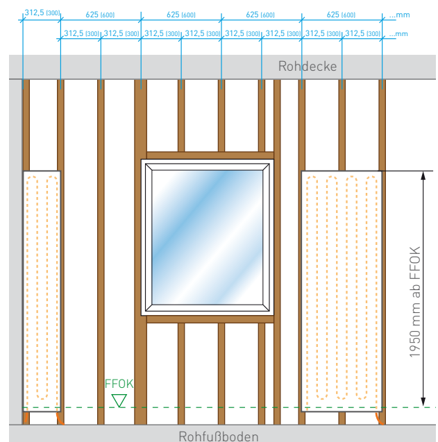
▲ Beispiel Holz-Ständerkonstruktion
