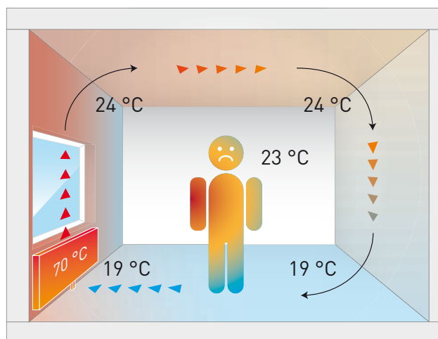
▲ Unbehaglichkeit mit Heizkörper
