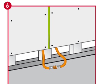
▲ Beispiel fertige Press-Kupplung bei bestehendem Boden (Sanierung)
