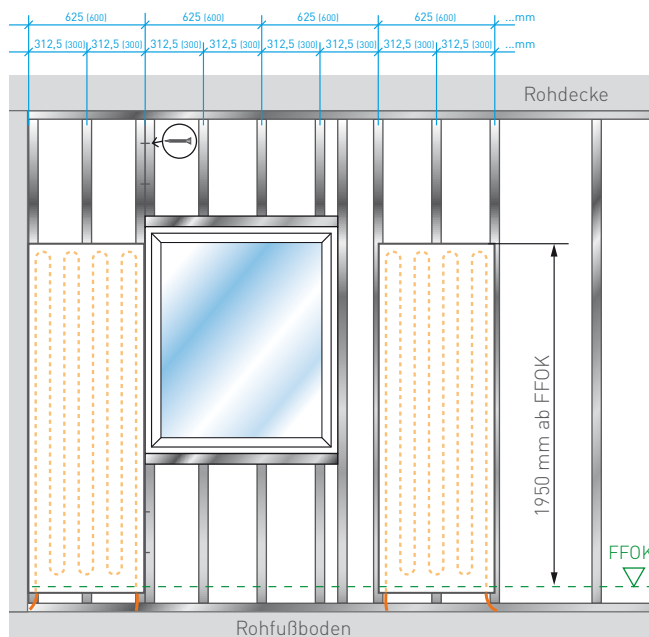
▲ Beispiel CW-Ständerprofilkonstruktion
