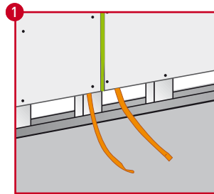
▲ Gequetschte Rohrenden rechtwinklig abschneiden
