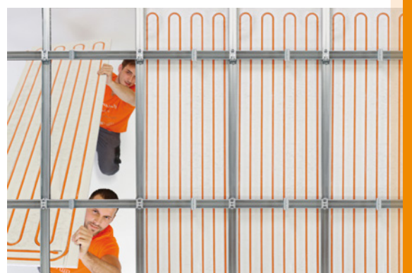
Montage
