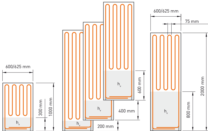
5 PLATTEN MIT VARIABLER HÖHE ModulDecke-Classic und ModulWand mit variabler Höhe
